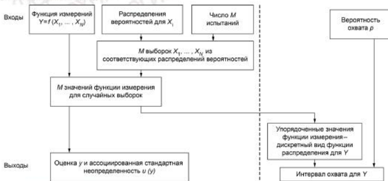
Рисунок 8 — Оценивание неопределенности методом Монте-Карло (левая часть рисунка, выделенная пунктирной линией, относится к получению значения оценки y и ассоциированной с ней стандартной неопределенности u(y) , остальная — к получению интервала охвата для Y )
