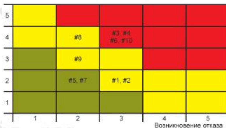
Рисунок С.3 — Матрица критичности для отчета FMECA в соответствии с таблицей С.5, разработанная в виде двумерного изображения, без учета обнаруживаемости
