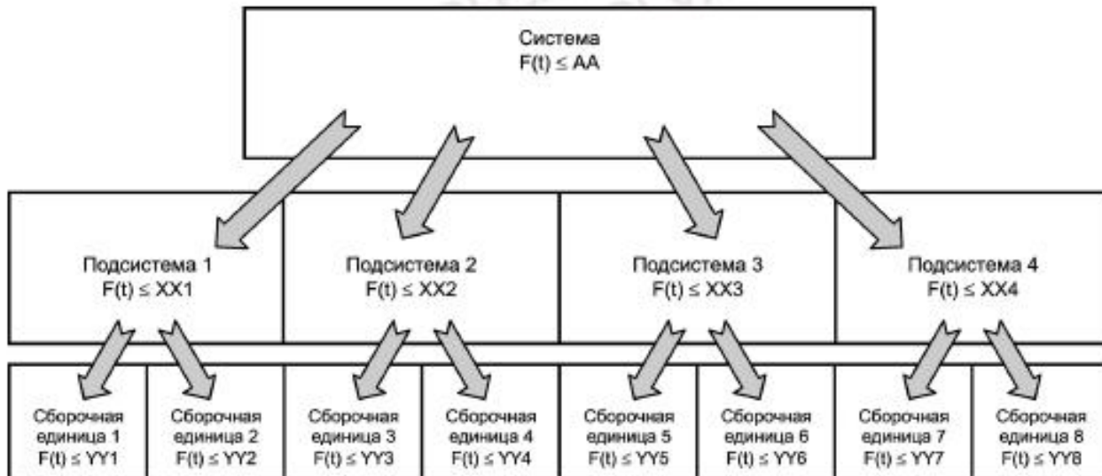
Рисунок Е.2 — Распределение вероятностей отказа в системе
