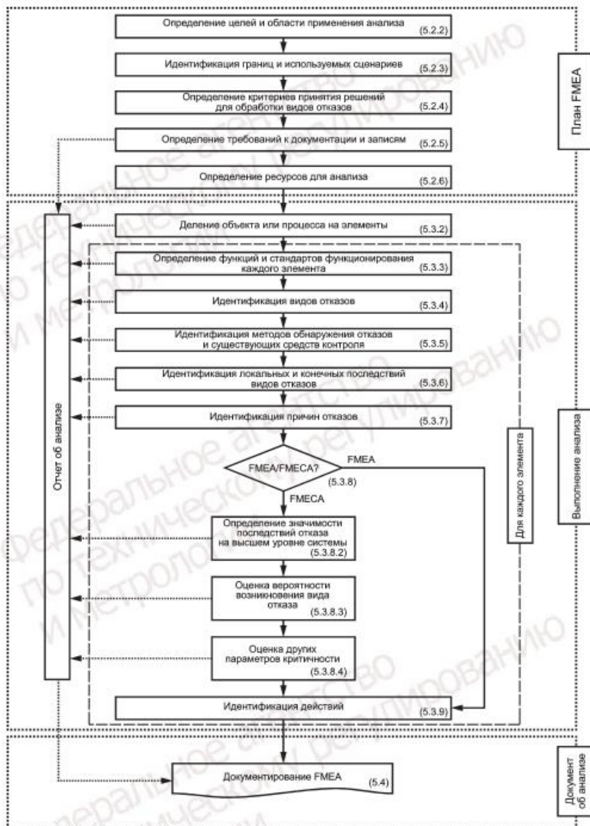
Рисунок 1 — Общая методология FMEA (до адаптации)
