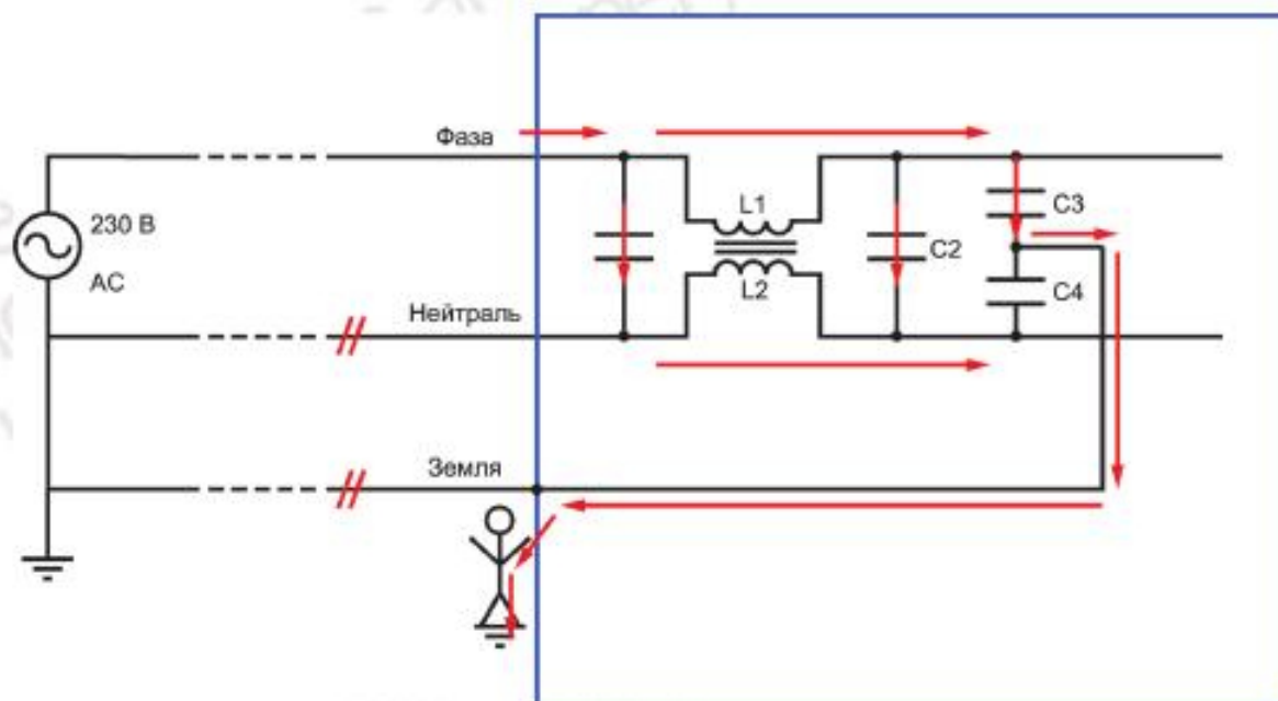
Рисунок С.2 — Схема источника питания типа XYZ
