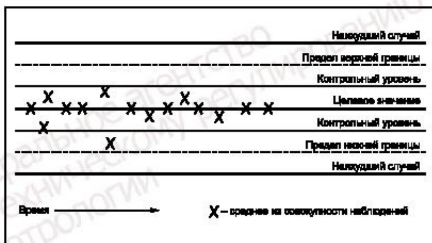
Рисунок А.9 — Контрольная карта
