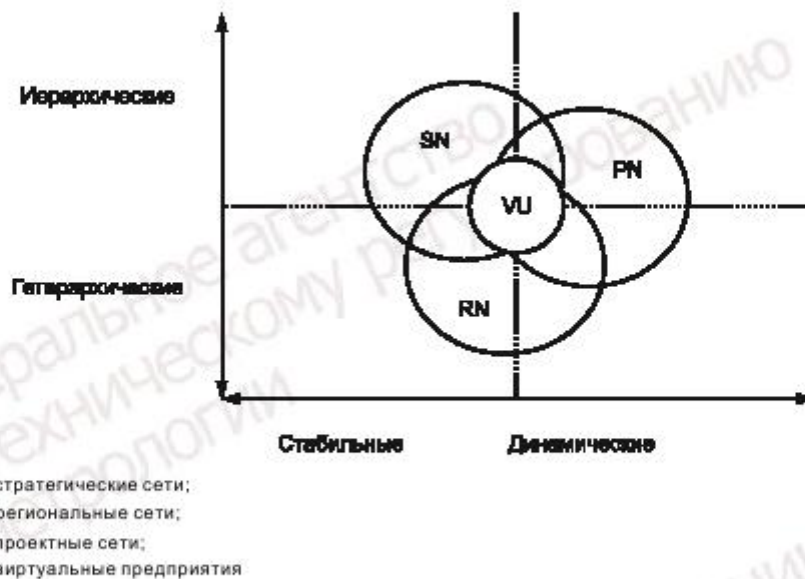
Рисунок 2 — Типологии сетей
