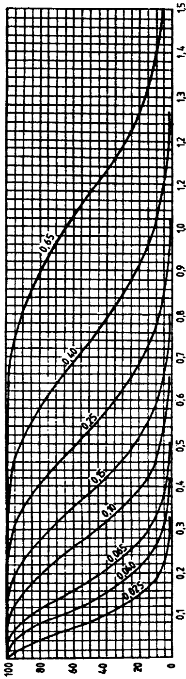
График R — Кривые оперативных характеристик для одноступенчатых планов (кривые двух- и многоступенчатого контроля по возможности максимально близки)
