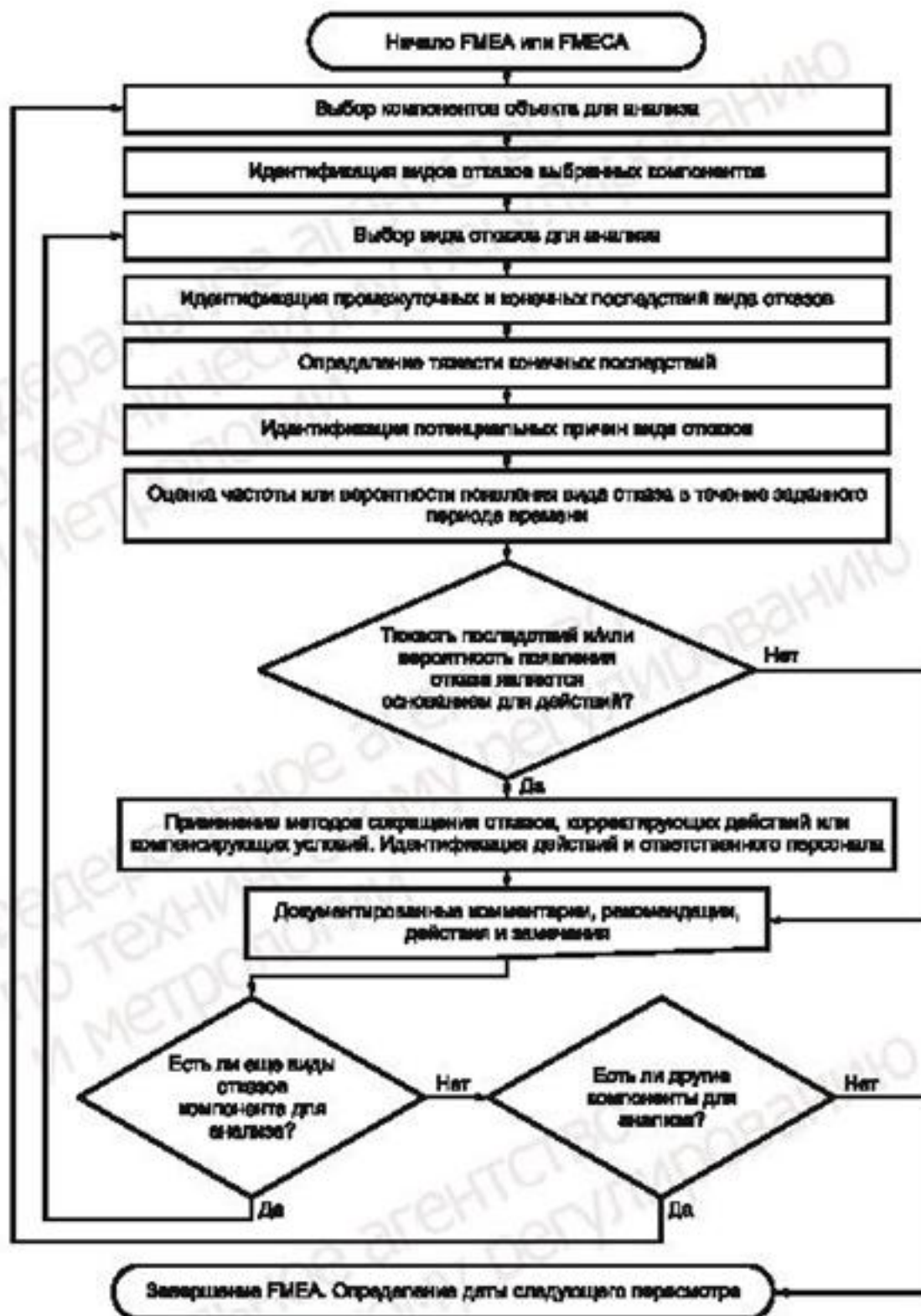
Рисунок 2 — Блок-схема анализа
