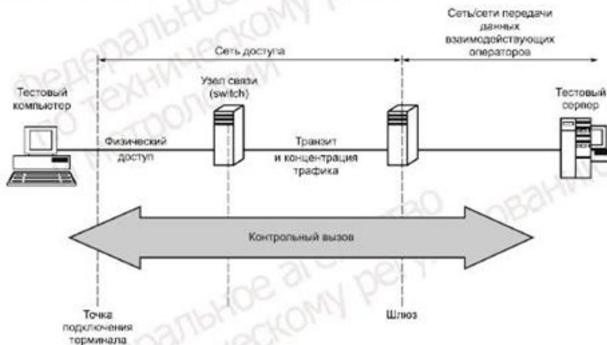
Рисунок Б.1 — Измерительная установка
