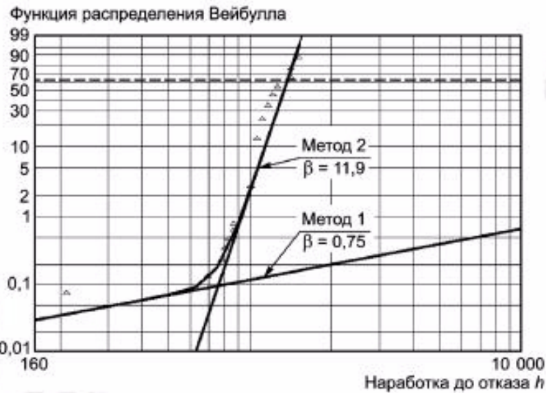
Рисунок А.2 — Отказы подшипников дополнительных насосов
