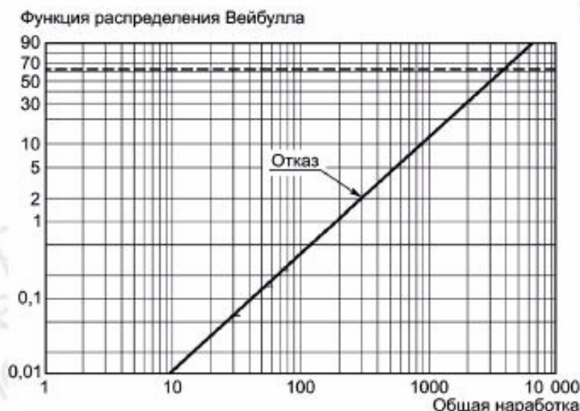
Рисунок А.1 — Ранние отказы масляных насосов
