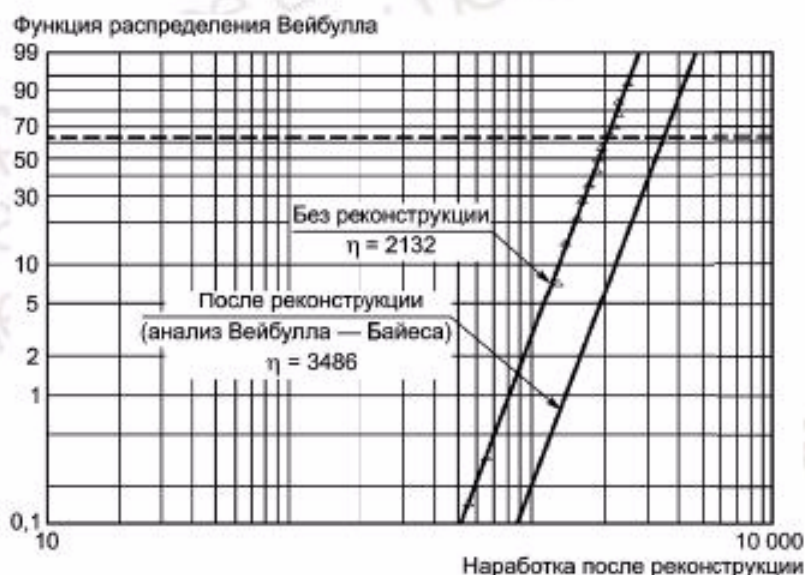
Рисунок 10 — Реконструированный компрессор и старый компрессор
