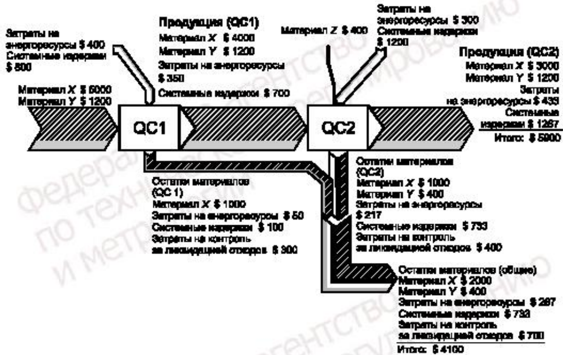
Рисунок В.4 — Диаграмма Сенки обобщенной информации
