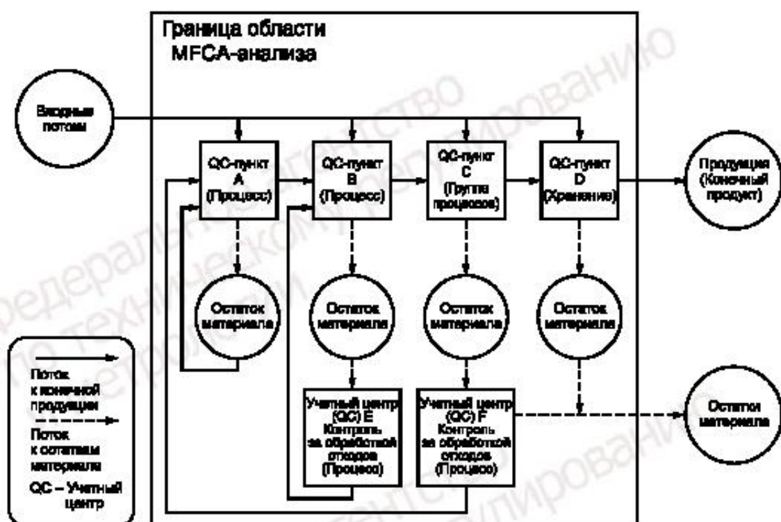
Рисунок 3 — Модель потока материала для процесса в пределах области MFCSA-анализа
