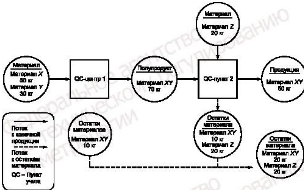
Рисунок В.2 — Модель потока материалов с учетом полупродуктов
