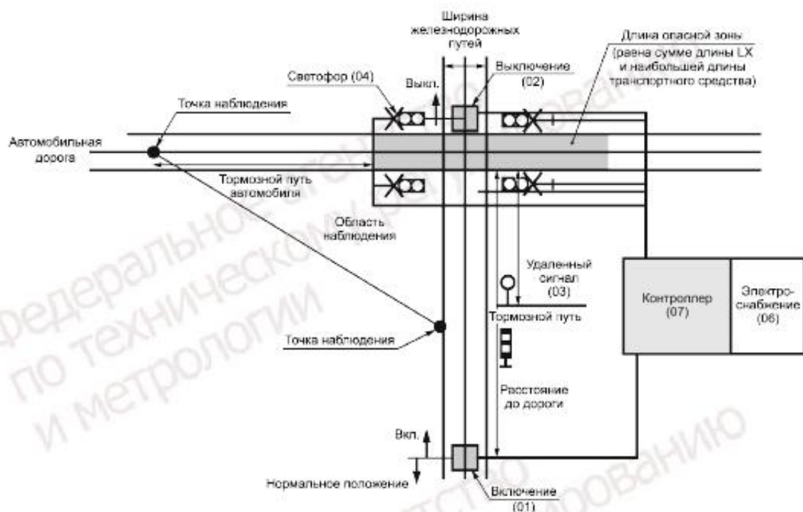
Рисунок В.3 — Система железнодорожного переезда (LX)
