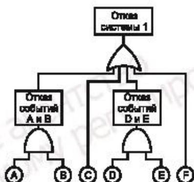
Рисунок В.6 — Дерево неисправностей для системы 1
