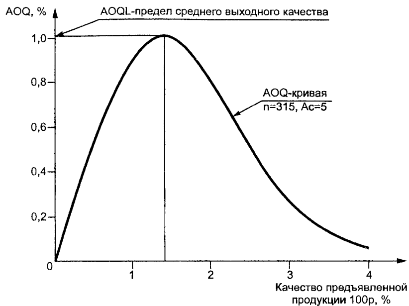
Рисунок 1 — AOQ и его предел AOQL
