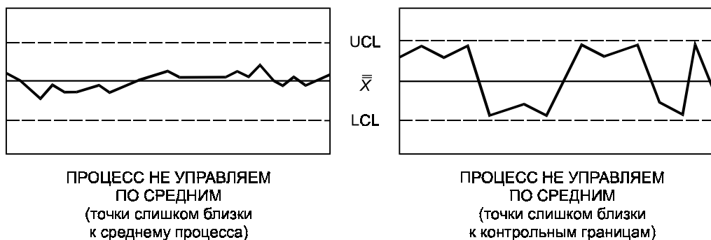
Рисунок 6 — \bar{X} -карта. Неслучайное поведение
