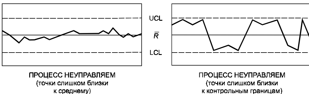
Рисунок 3 — R-карта. Неступное поведение данных процесса
