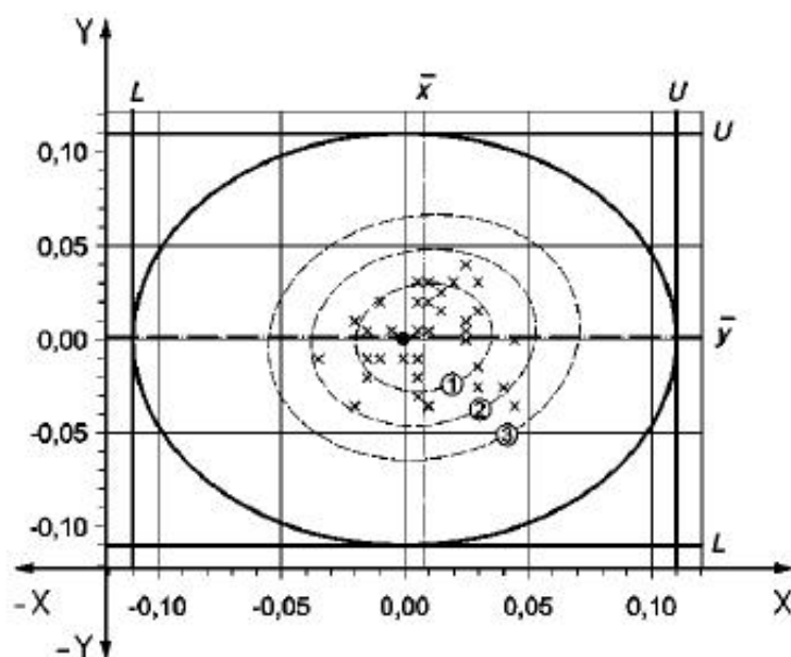
Рисунок 7 – Зона допуска для позиционного допуска
