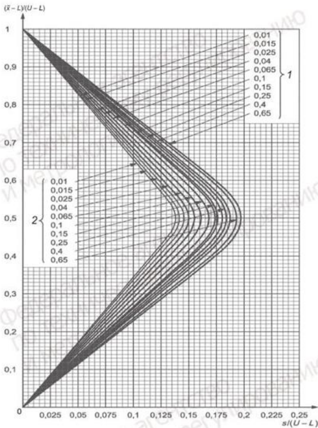
Рисунок 32 — График z-R. Приемочные кривые для объединенного контроля с двумя пределами поля допуска и общим AQL. «z» метод. Код объема выборки R (объем выборки 250)
