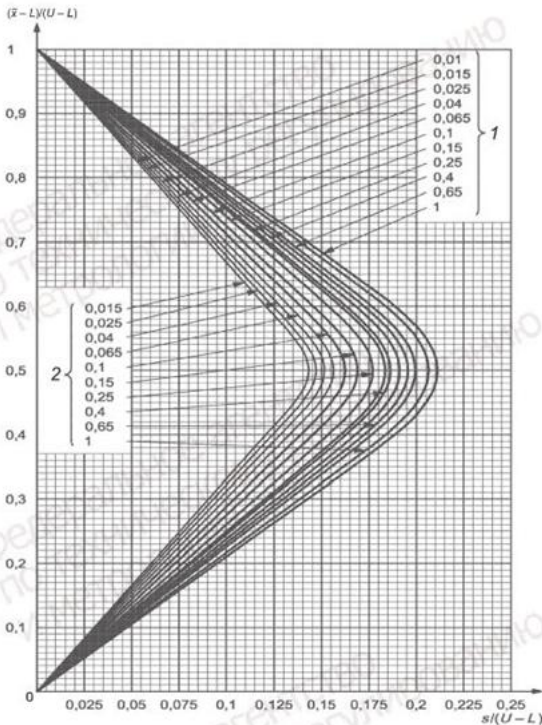
Рисунок 31 — График s-Q. Приемочные кривые для объединенного контроля с двумя пределами поля допуска и общим AQL. «в» метод. Код объема выборки Q (объем выборки 200)
