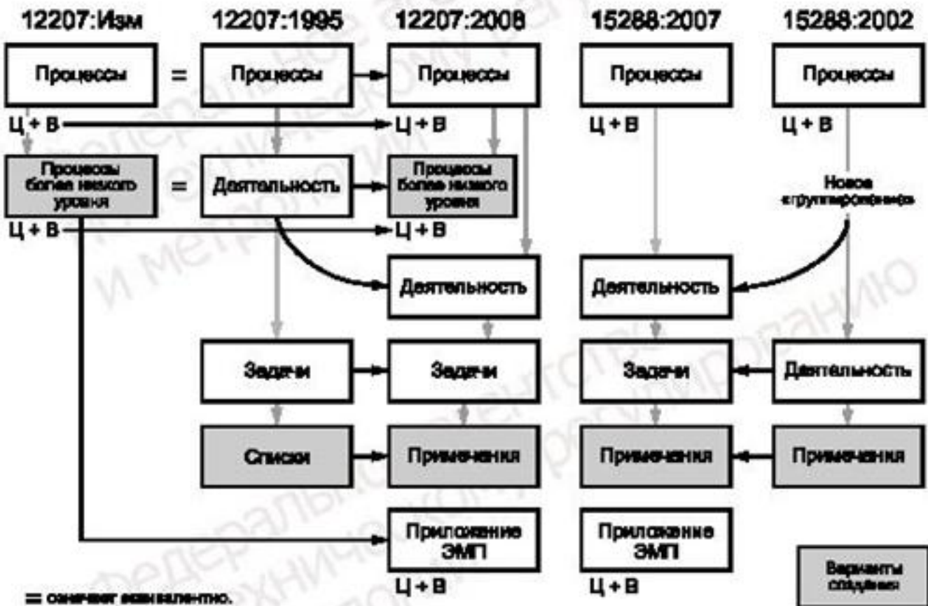
Рисунок С.2 — Отношения между конструкциями процессов
